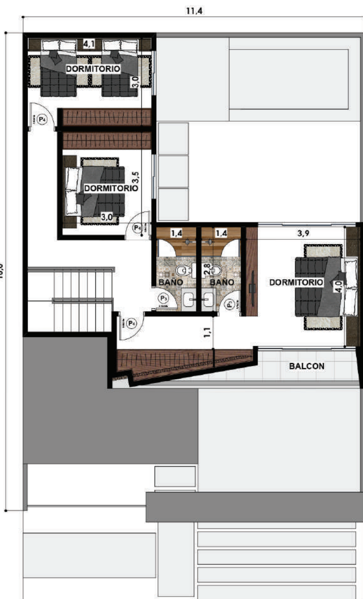
PLANTA ALTA
